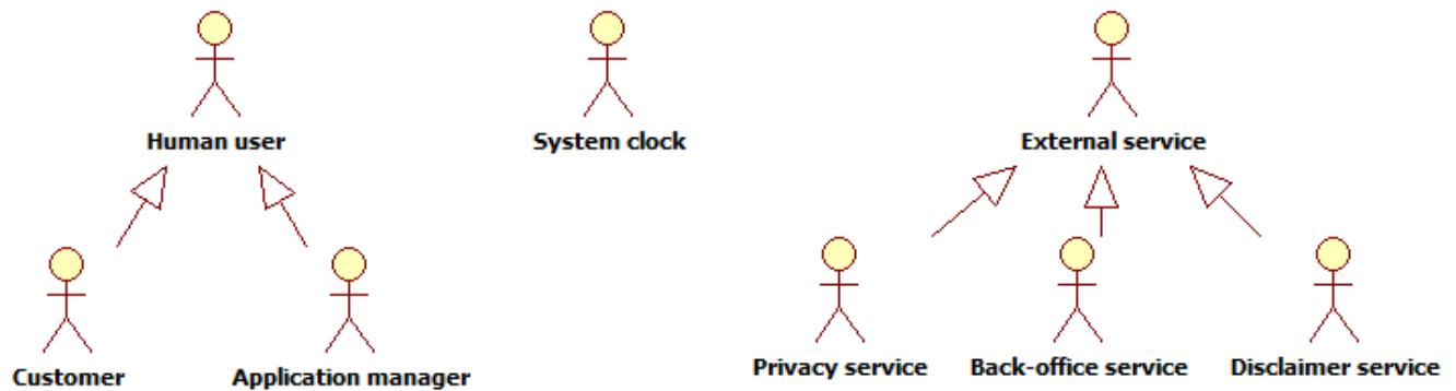
Figura 9 - Attori del sistema
