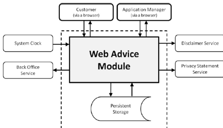
Figura 27 - Confine nel "Web Advice Module"
