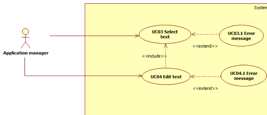
Figura 12 - Use case Manutenzione - Select Text & Edit Text
